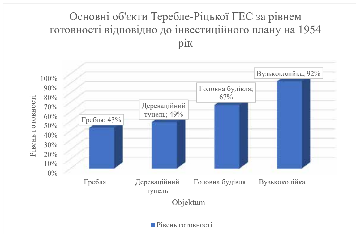
Рис. 3. Основні об'єкти Теремле-Ріцької ГЕС за рівнем готовності відповідно до інвестиційного плану на 1954 рік
